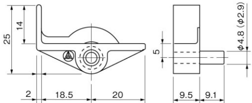
差込み棚ダボGM
