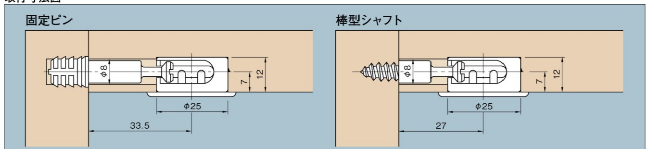
取付寸法図
