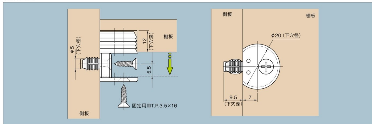
取付寸法図
