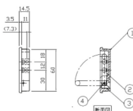
ビス穴断面詳細図 S2/1
